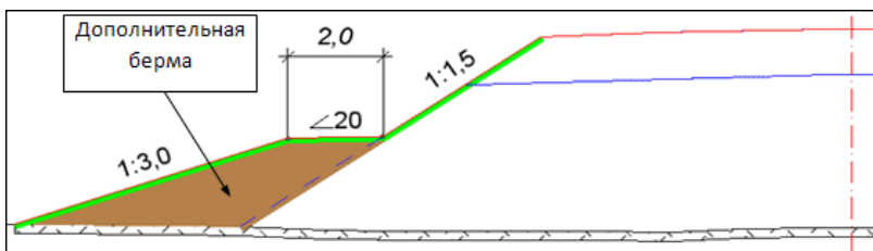
* Насыпь с дополнительной бермой на расчетной высоте.
