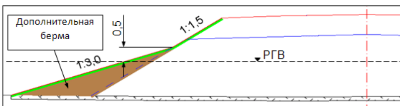
* Насыпь с измененной крутизной откосов на расчетной высоте.
